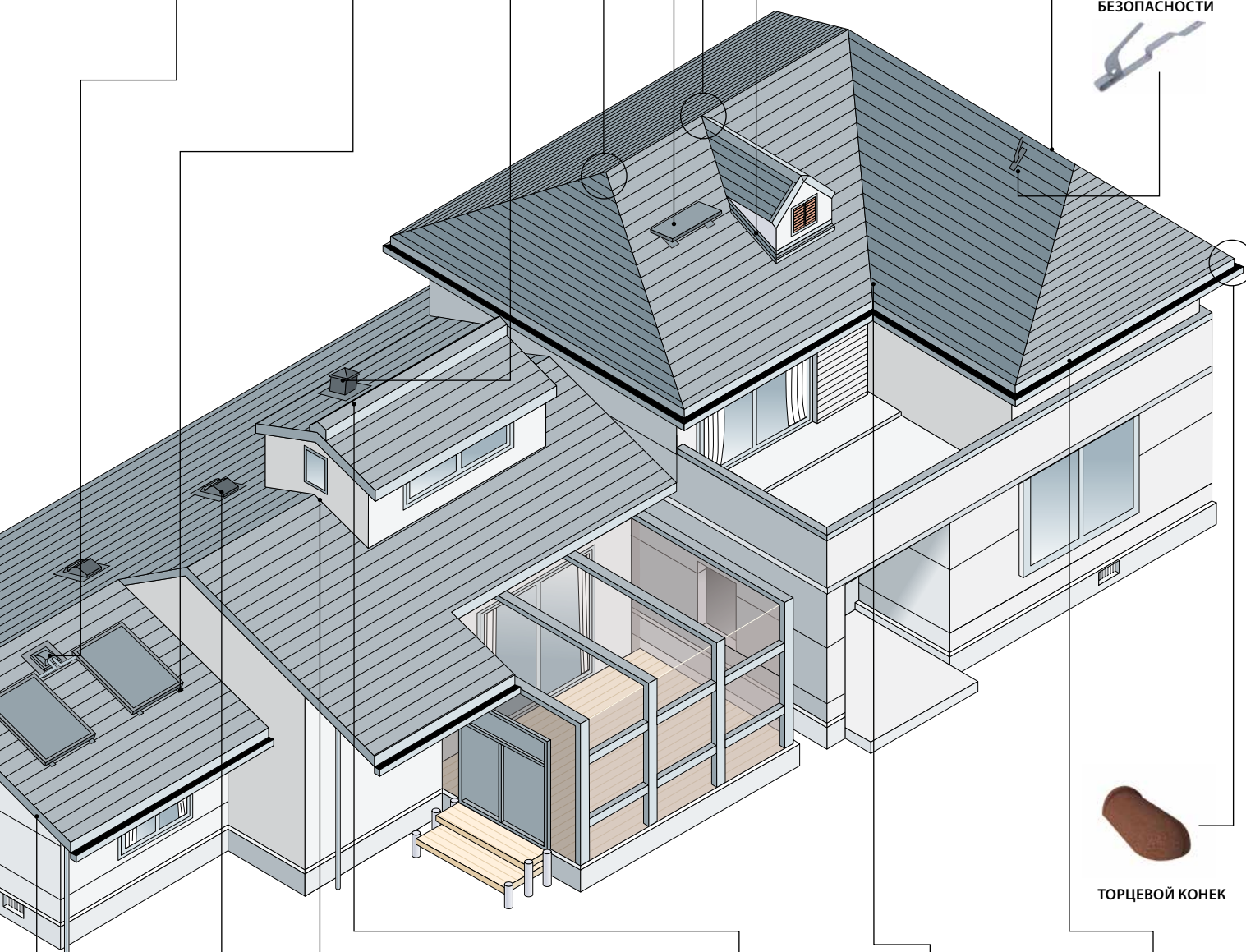
КРЮК БЕЗОПАСНОСТИ
